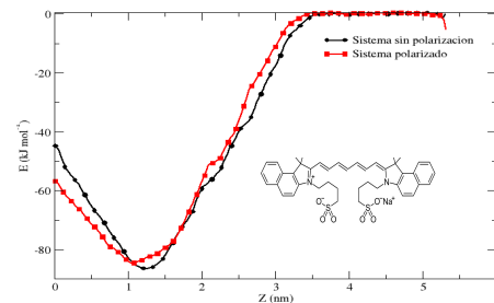
Fig.1 : Inserción de un colorante sensible al voltaje en una bicapa lipídica. La curva roja representa el perfil de energía libre de partición. Inserto: estructura molecular de ICG.
